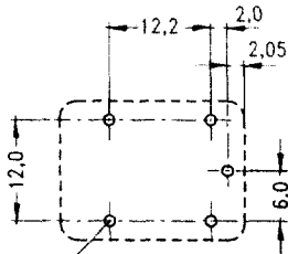
All holes \varnothing 1,3 mm
